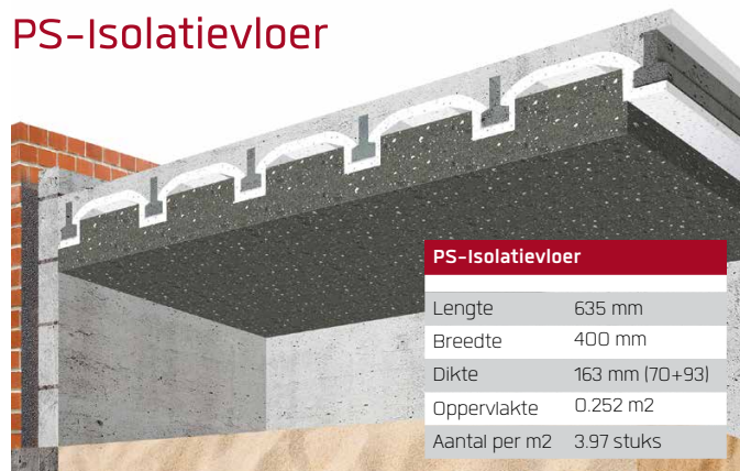
PS-insulatievloer met Easy Inserts Rc-waarde totale vloerconstructie = 4,81 m2K/W
